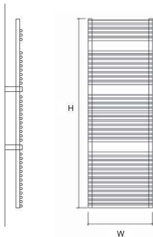
H170 - 37 tubes
